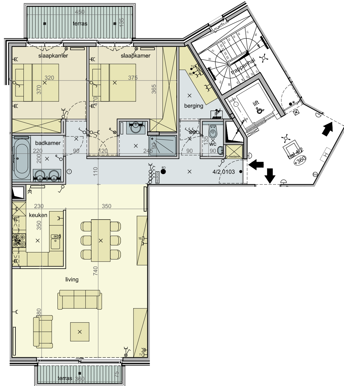
1e verdieping appartement 4/2 0103, schaal 1/100
